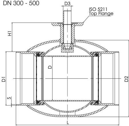
DN 300 - 500
